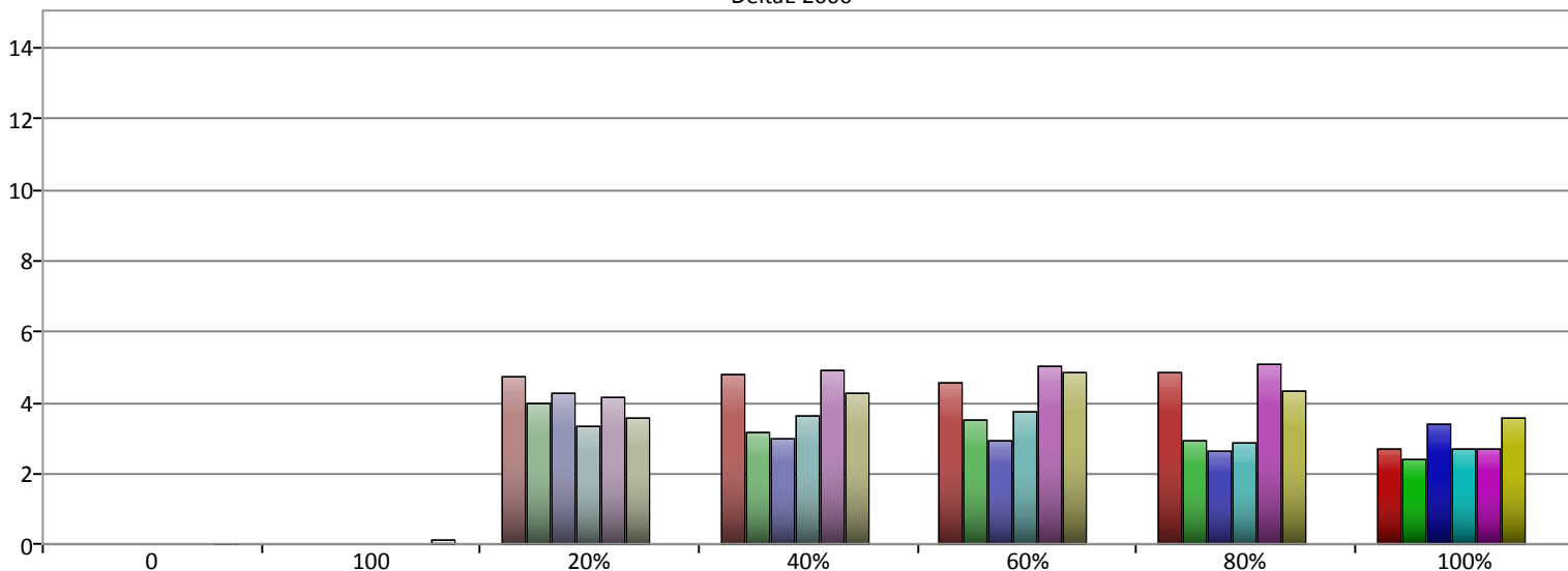
DeltaE 2000
